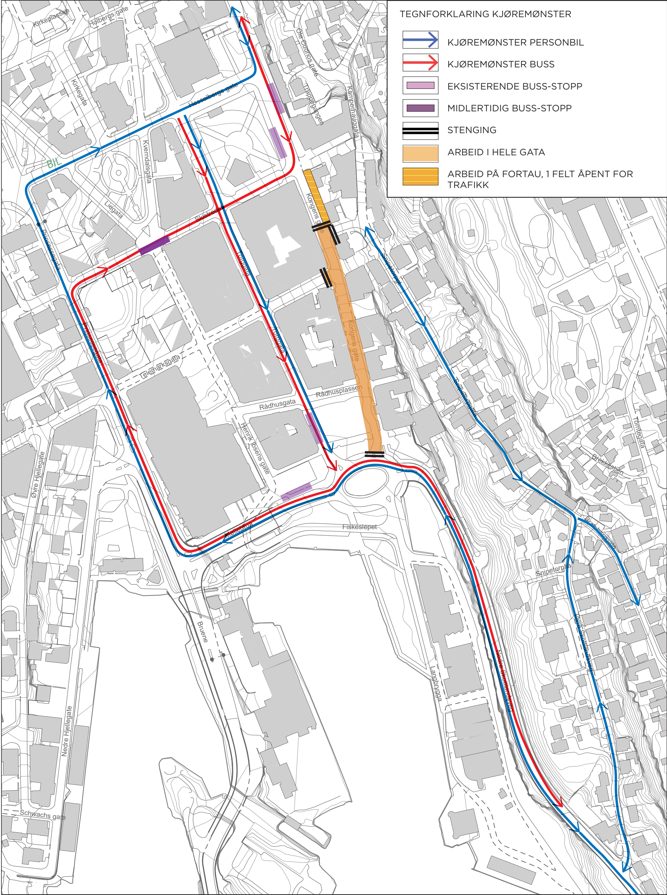
Oppgradering av Kongens gate Trafikkavviklingsplan fase 6 Gyldig fra 15/10 - 25
