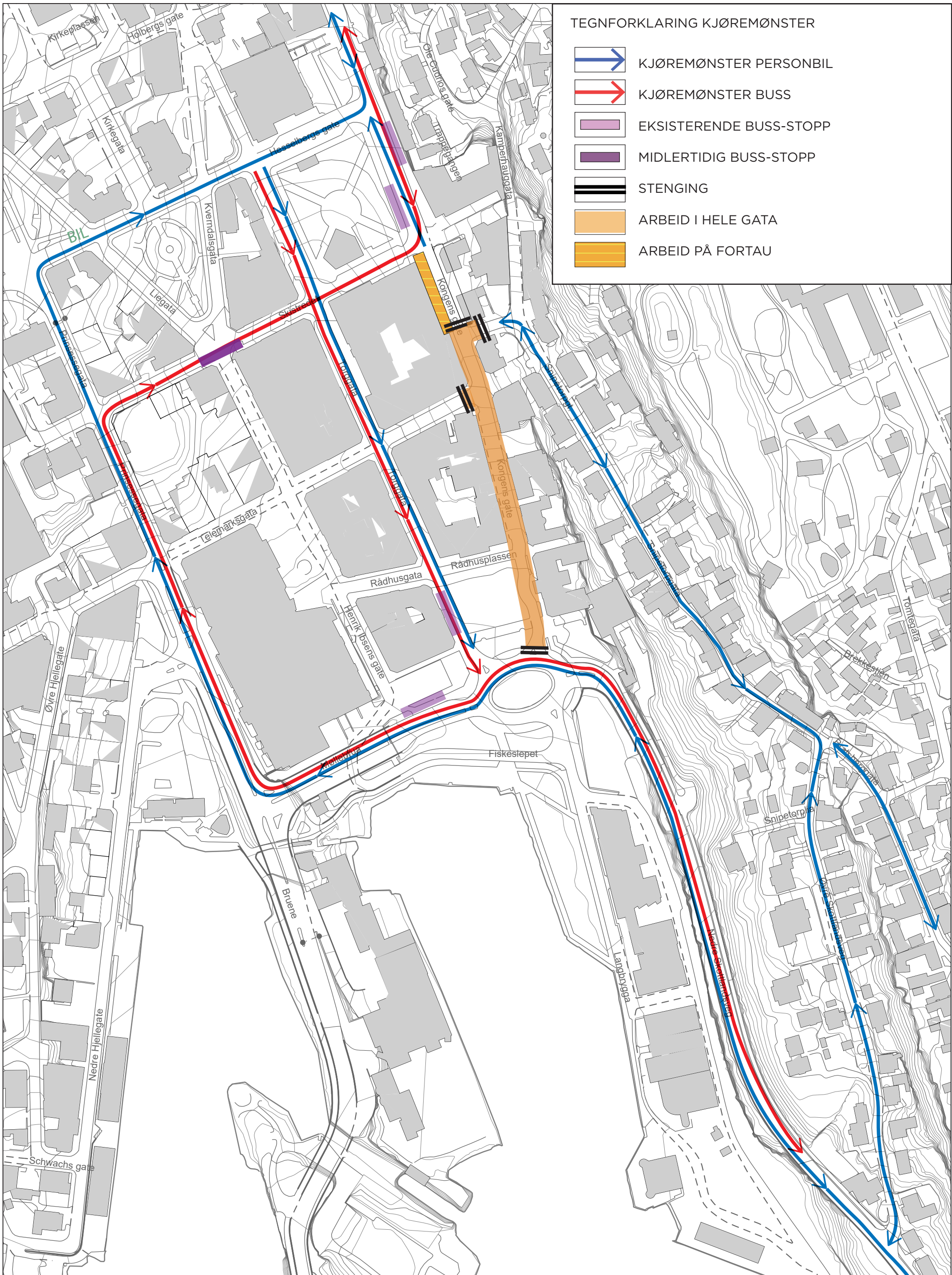
Oppgradering av Kongens gate Trafikkavviklingsplan fase 3 (rev 1) Gyldig fra 7/7-25
